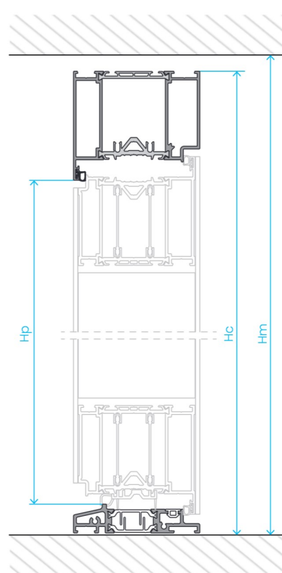
Przekrój pionowy
