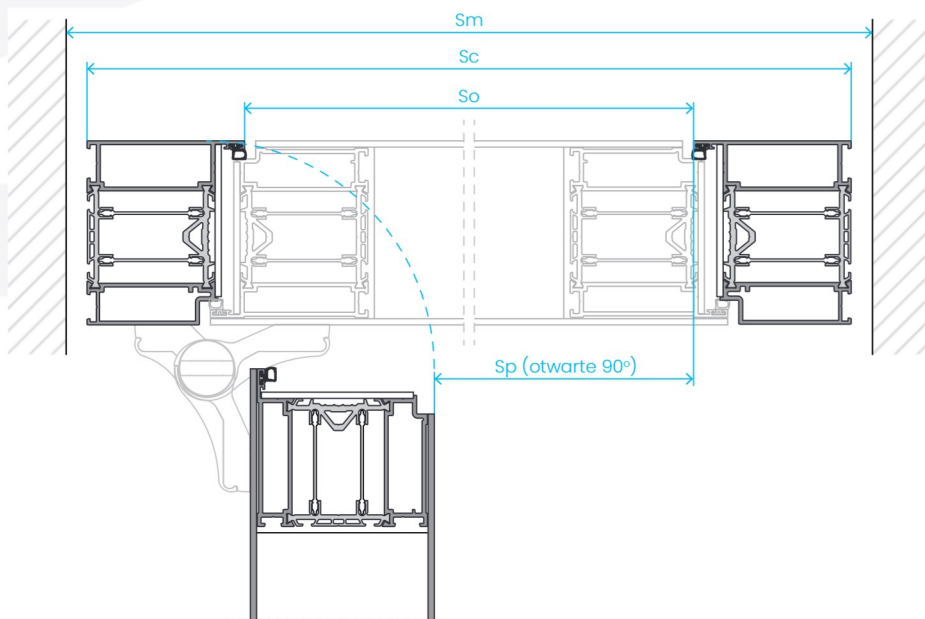
Przekrój poziomy
